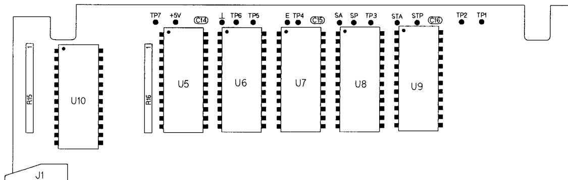
Figure B-4. 08116-66533: ROM layout
